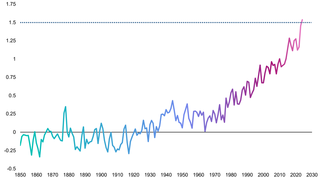
Global mean temperature 1850-2024 (°C)
